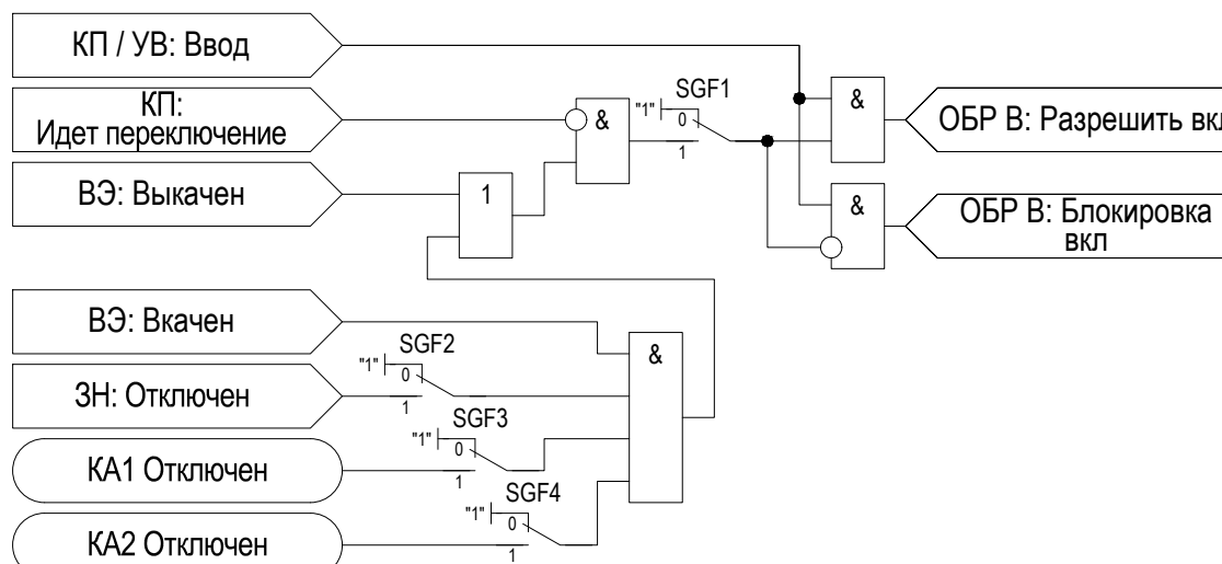
Рисунок 2.59 – Функциональная схема «ОБР В»
