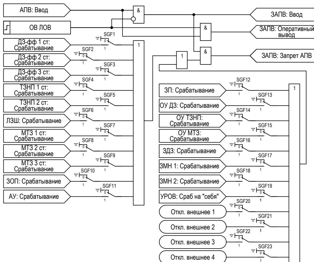
Рисунок 2.51 – Функциональная схема «ЗАПВ»
