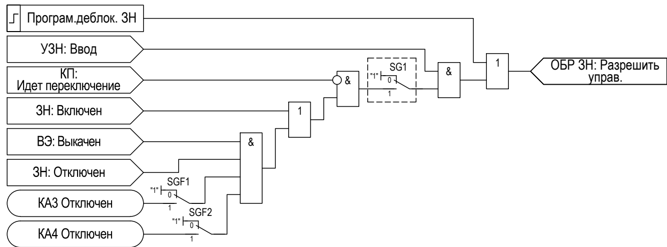
Рисунок 2.61 – Функциональная схема «ОБР ЗН»
