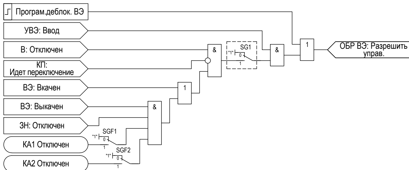
Рисунок 2.60 – Функциональная схема «ОБР ВЭ»
